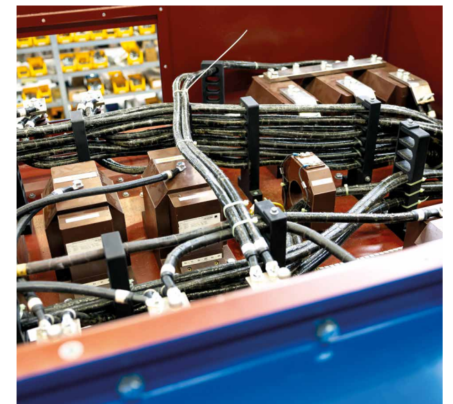
Boîte à bornes principale en détail
